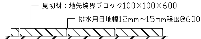
A-A断面図
